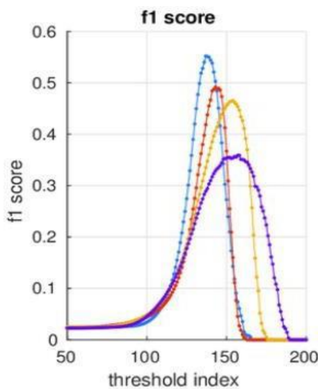
Fig.19. F1 Score.
