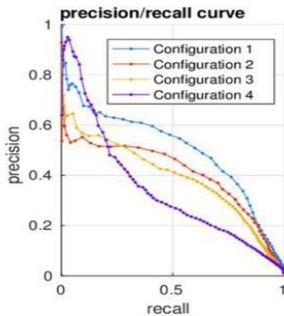
Fig.18. Precision/Recall curve.
