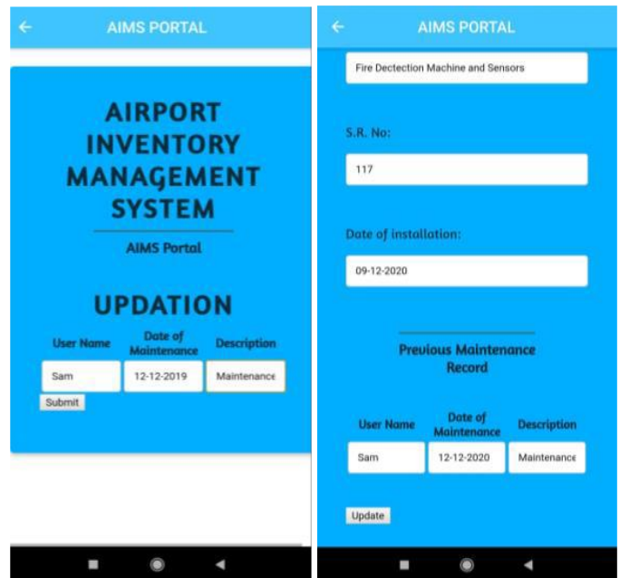
Fig. 10. Updation Page
