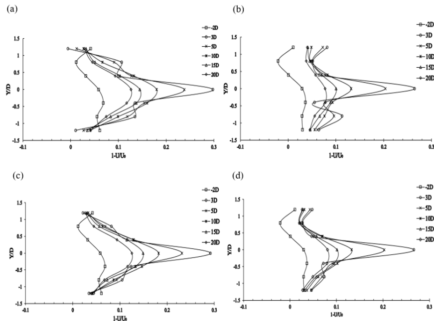
Figure 6 : Lateral variation of velocity deficit in (a) E3,1.5, (b) E3,2, (c) E6,1.5, (d) E6,2
