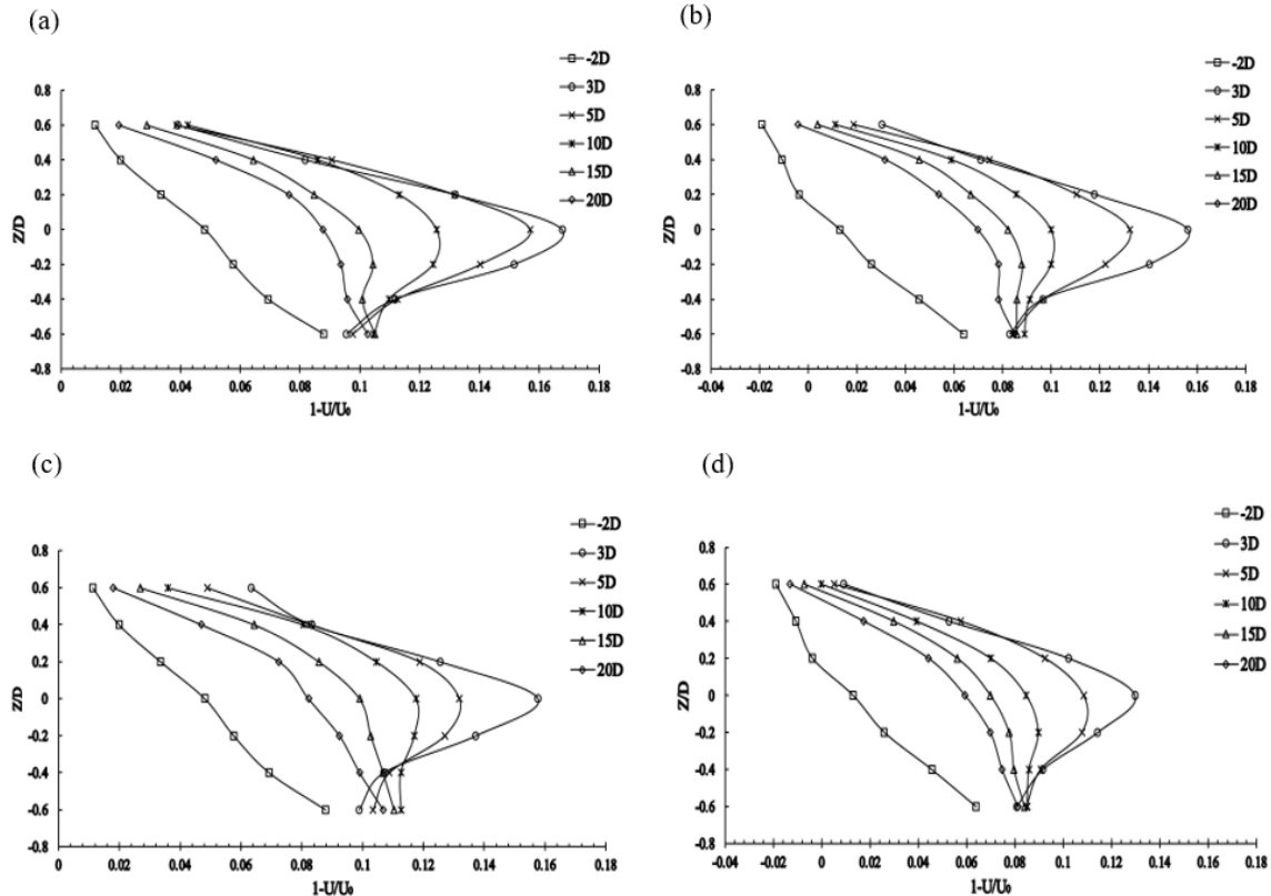
Figure 4: Vertical profile of velocity deficit (a) E3,1.5, (b) E3,2, (c) E6,1.5, (d) E6,2
