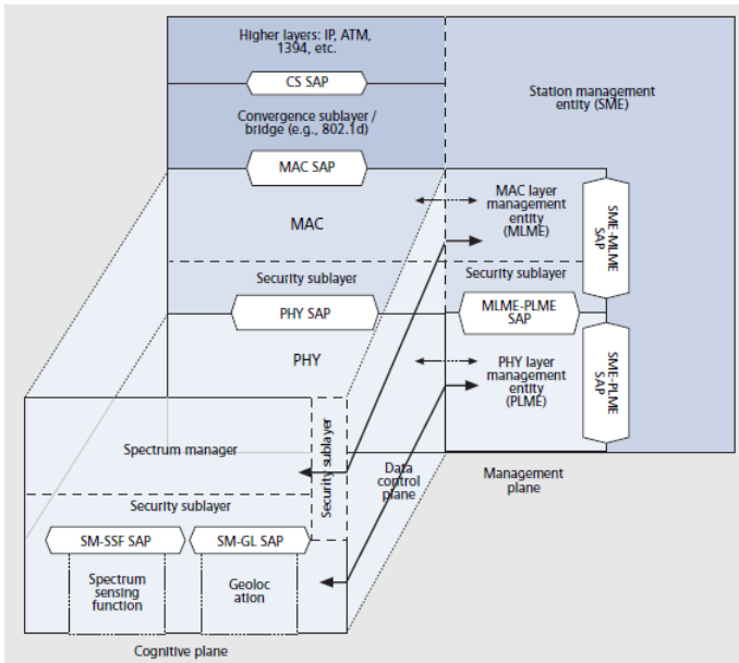
Figure 15. CR interface : IEEE 802.22
