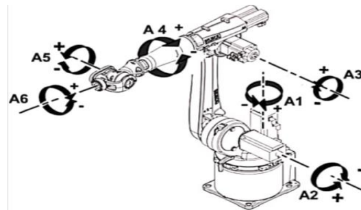
Fig. 4. Kuka Robot
